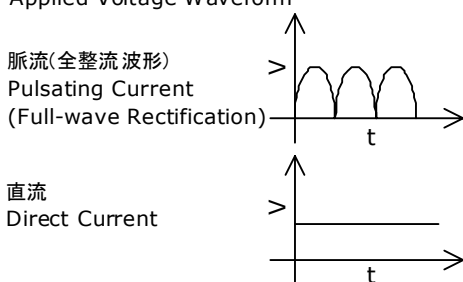
** 印加電圧波形 Applied Voltage Waveform
